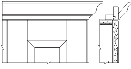
LM8+TMM8 H ADJ: 2-3/4" ~ 3-3/4"
