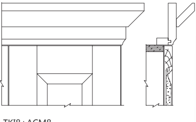
TKI8+ACM8 H ADJ: 4-1/2" ~ 6"
