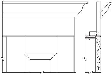
F696+TMM8 H ADJ: 6" ~ 7-1/2"
